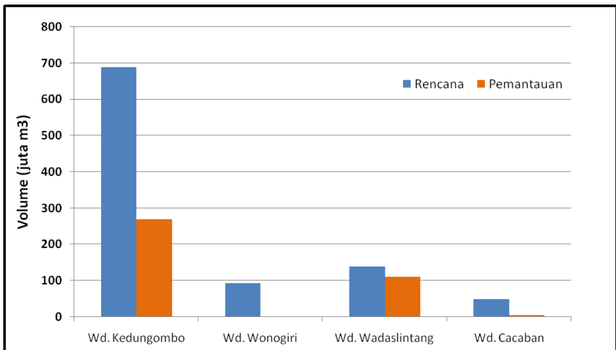
Gambar 4. Perbandingan Volume Rencana dan Pemantauan 4 Waduk Utama di Jawa Tengah (Status 01 s/d 15 Oktober 2019)
