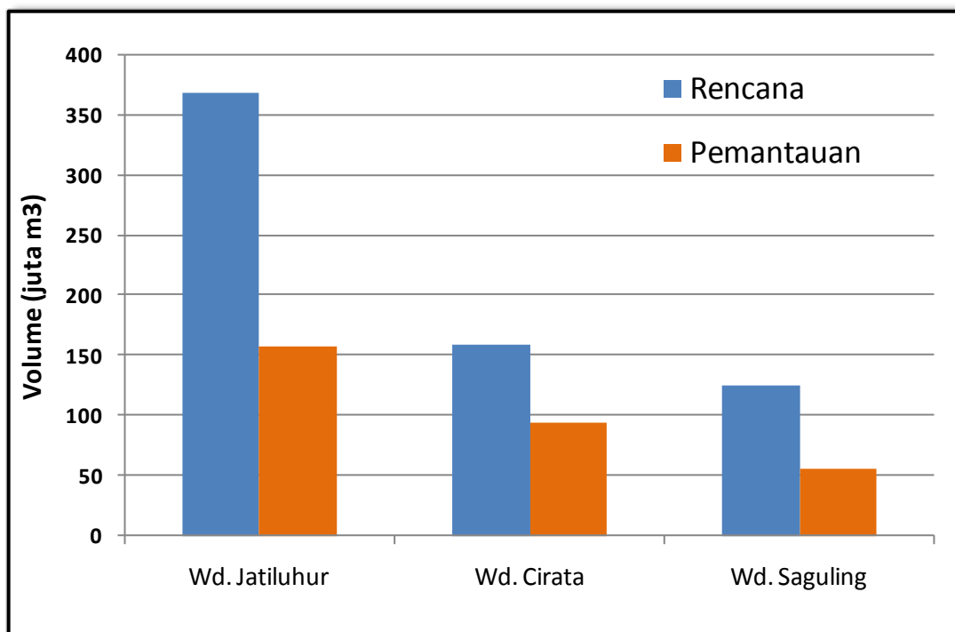
Gambar 3. Perbandingan Volume Rencana dan Pemantauan 3 Waduk Utama di Jawa Barat (Status 01 s/d 15 Oktober 2019)
