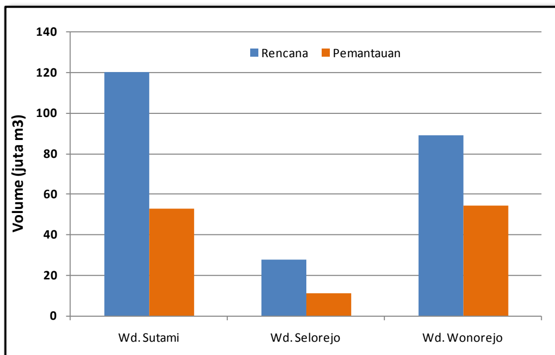
Gambar 5. Perbandingan Volume Rencana dan Pemantauan 3 Waduk Utama di Jawa Timur (Status 01 s/d 15 Oktober 2019)
