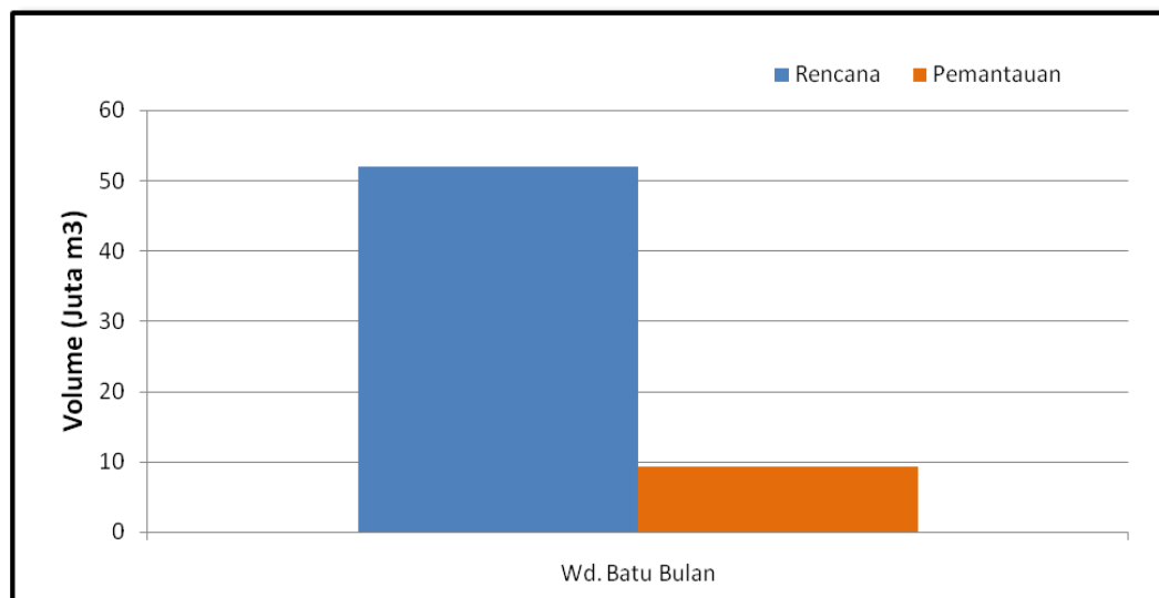
Gambar 7. Perbandingan Volume Rencana dan Pemantauan Waduk Batu bulan di NTB (Status 01 s/d 15 Oktober 2019)
